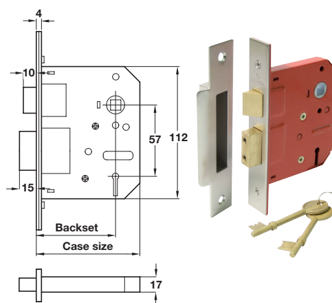
911.02.308 5 Lever mortice lock
