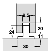
Bottom guide
