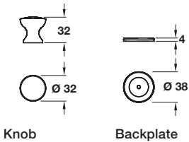
Knob Backplate
