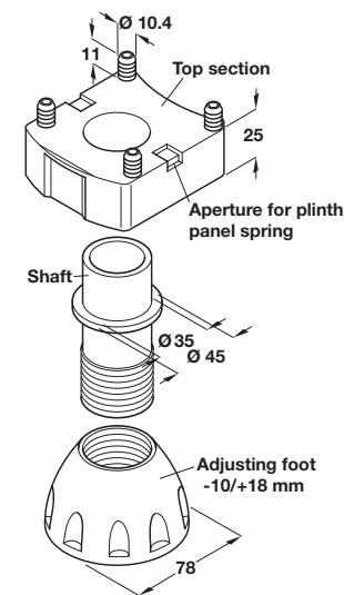
Press fit
