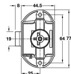
Push button espagnolette lock, 25 mm backset
