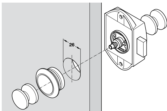
Push button espagnolette lock, 25 mm backset
