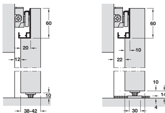
Door clearance 12 mm
