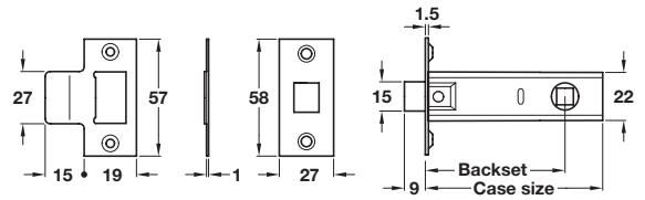
911.03.194 Tubular mortice latch
